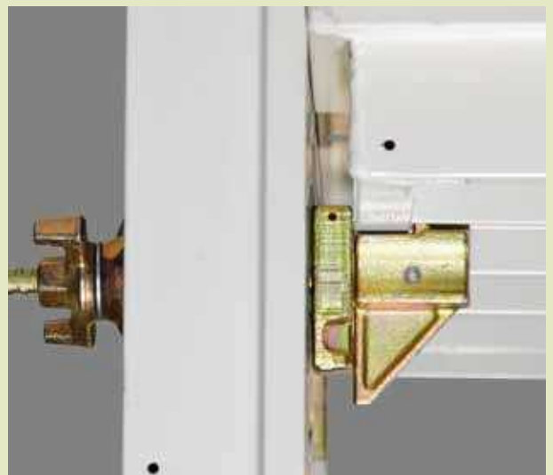
Klemme Ecke-Säule Morsa angolo-pilastro
