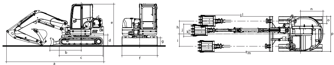
DIMENSIONI (mm)
