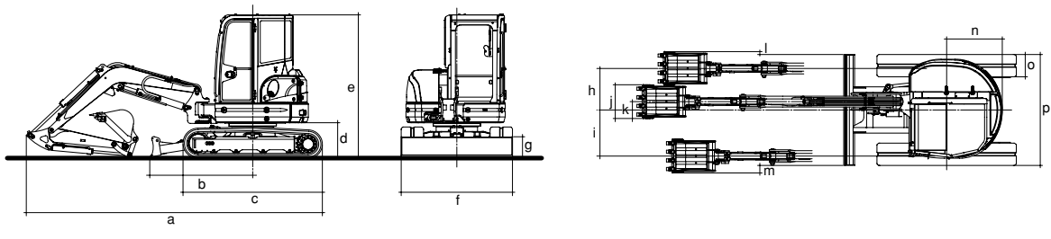
DIMENSIONI (mm)
