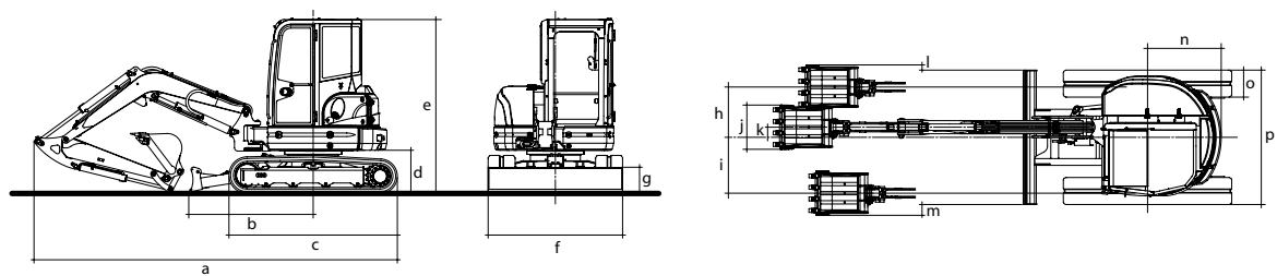
DIMENSIONI (mm)
